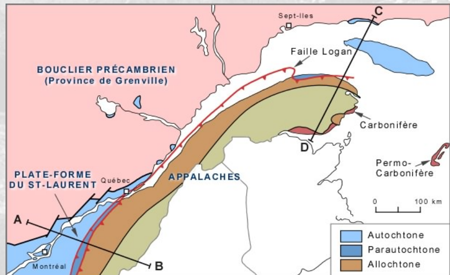
Figure 2. Les provinces géologiques du sud du Québec
